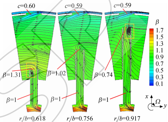
图7 不同管长下盘腔内的流线及旋流数云图
