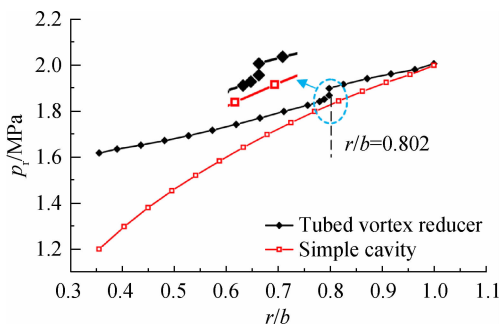
图6 简单盘腔与导流管盘腔内静压分布
