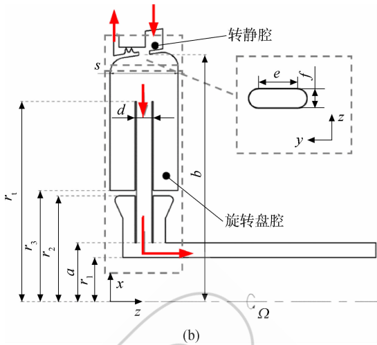
图 1 CFD 计算模型
