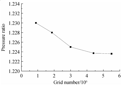
图 3 网格量的影响 Fig. 3 Influence of the grid number
