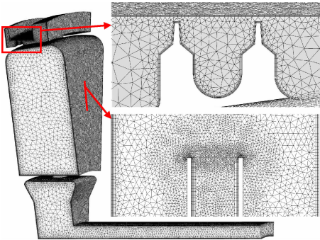
图 2 计算用网格示意 Fig. 2 Computational grids
