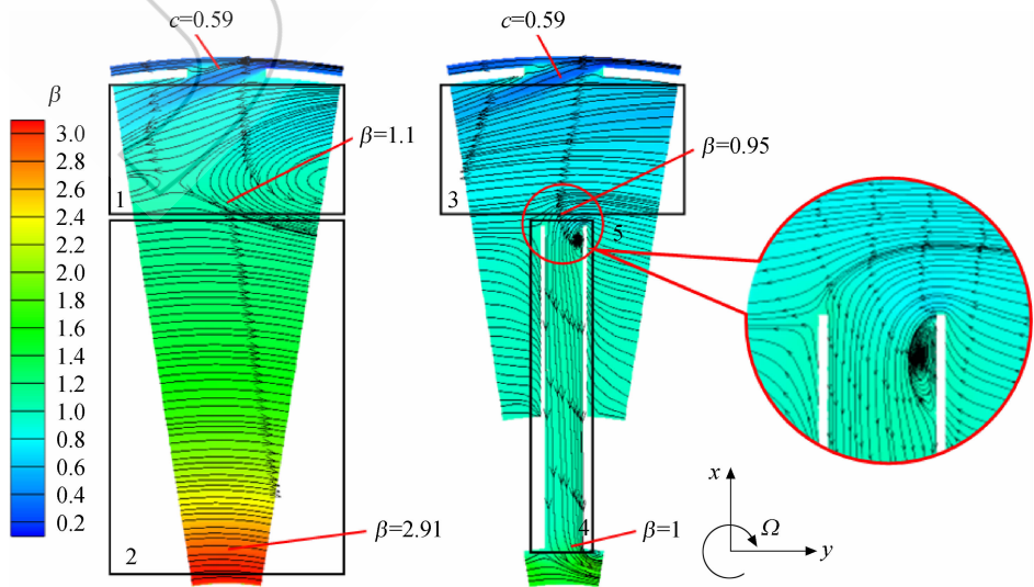
图 5 简单盘腔与导流管盘腔内流线与旋流数云图
